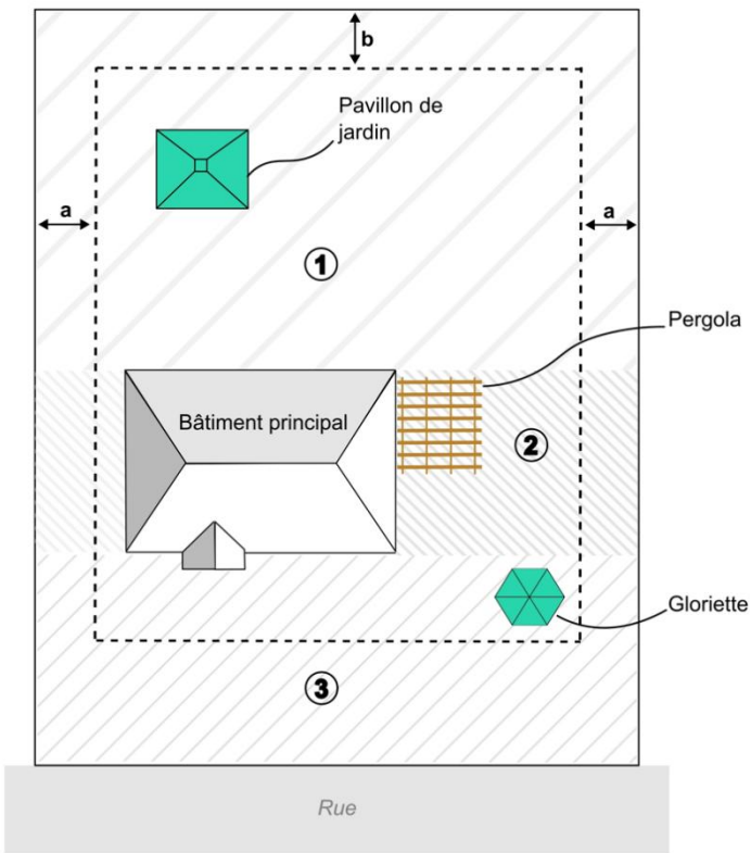
Croquis 6 : Implantation d'une gloriette, d'un pavillon de jardin et d'une pergola
