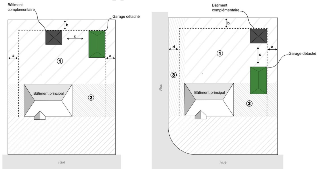
Croquis 5 : Garage détaché
